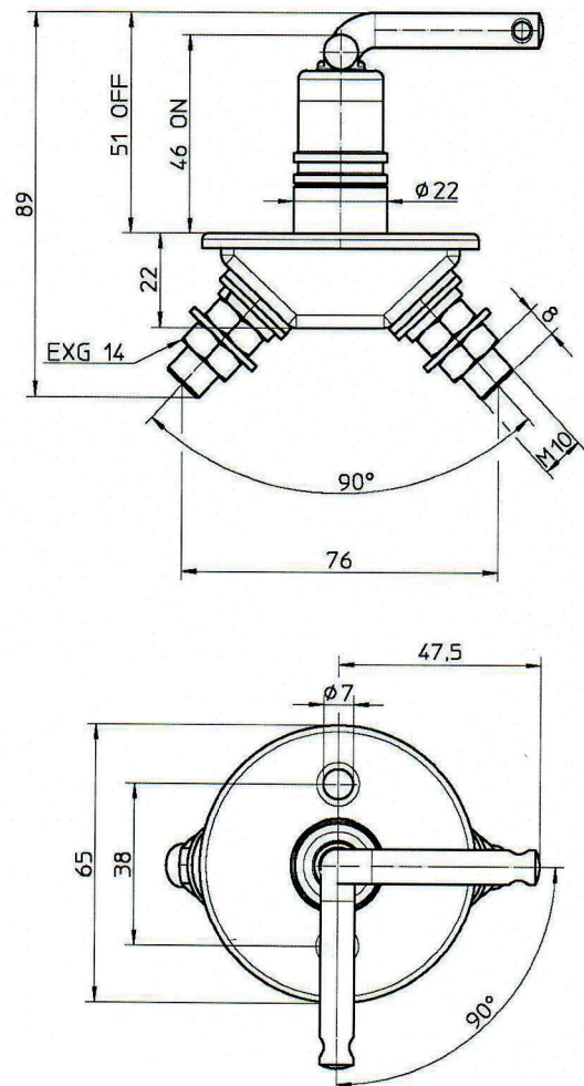
Esquema dimensional
